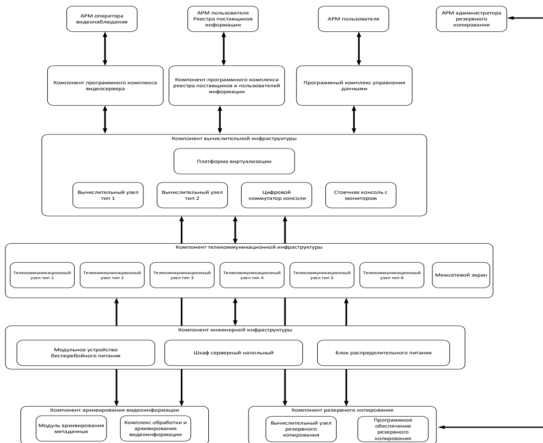
Рисунок 1. Схема функциональной структуры ПК «Периметр. Система видеонаблюдения»
